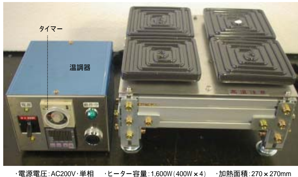
製作例-2・プレートヒーター・4枚タイプ(・タイマー/ブザー/表示灯付属)
