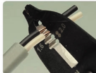
芯線ストリップ穴
